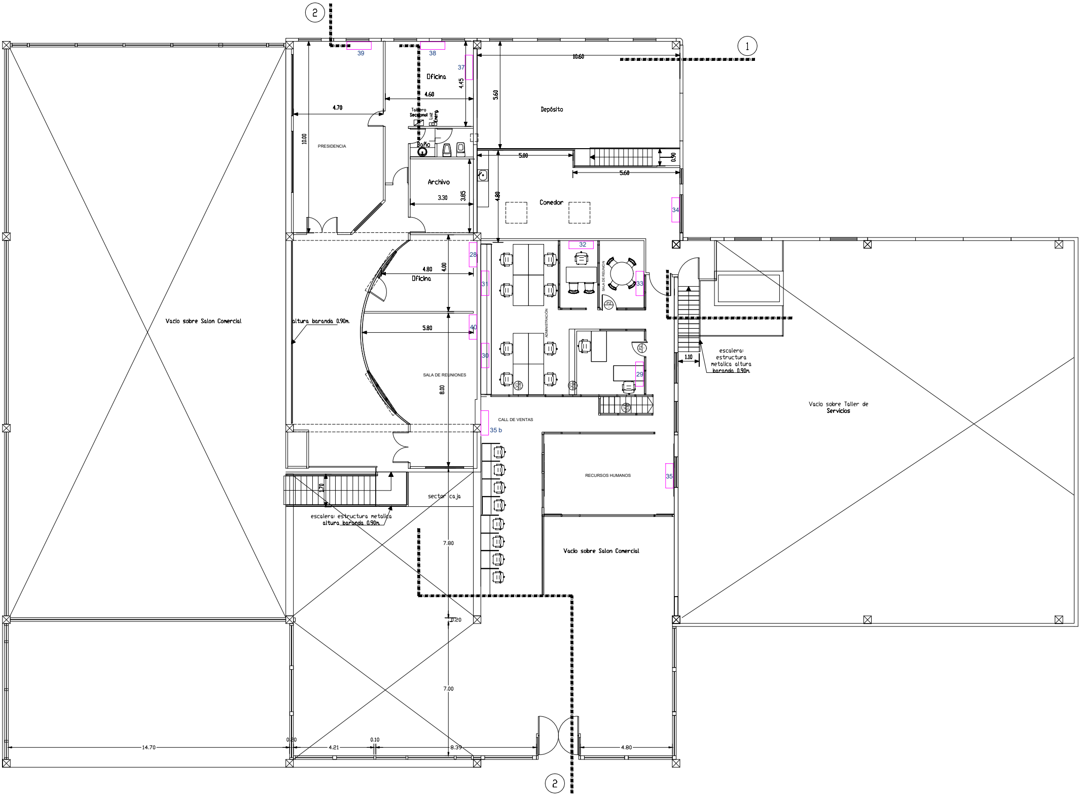
PLANTA ALTA TOYOTA COLON
